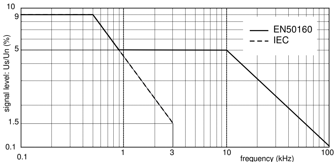
Fig 15b: Limites de tension des signaux du réseau selon les normes EN50160 et IEC
