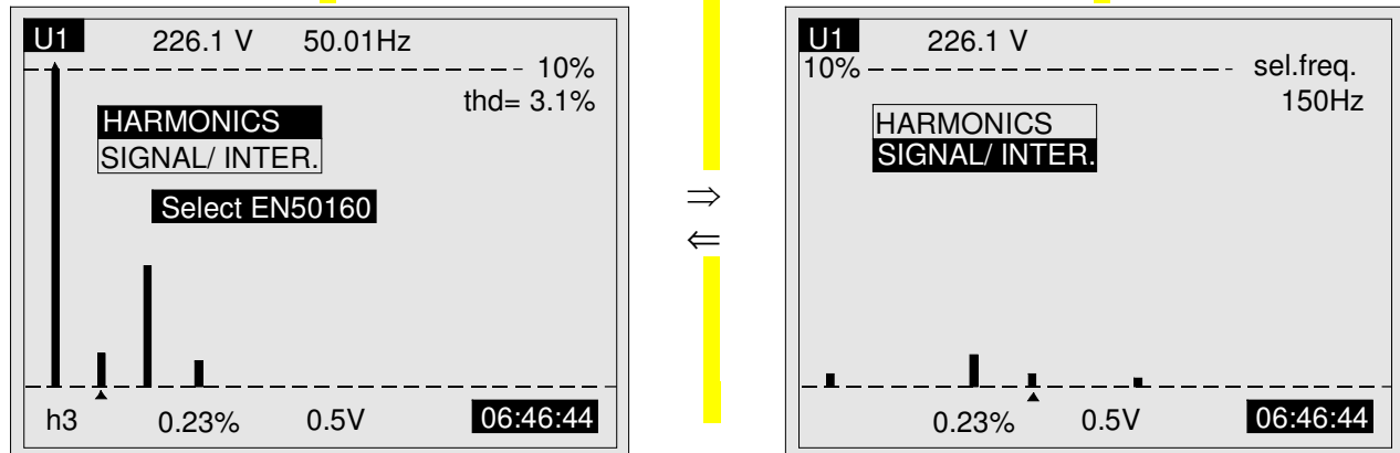
Fig. 15c: Signaux du réseau / Analyse interharmonique
