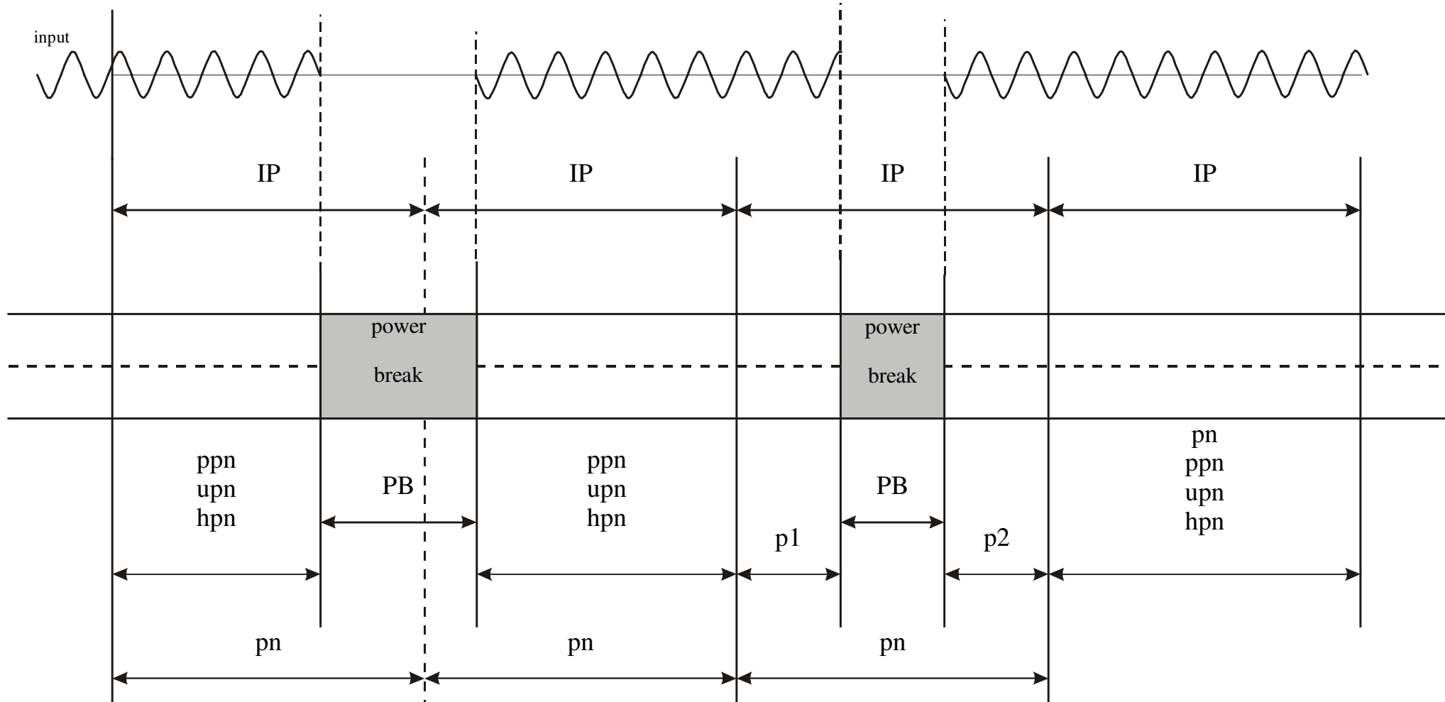
Fig. 48: Cycles d'entrée utilisés pour le calcul dans des situations de rupture de courant variées
