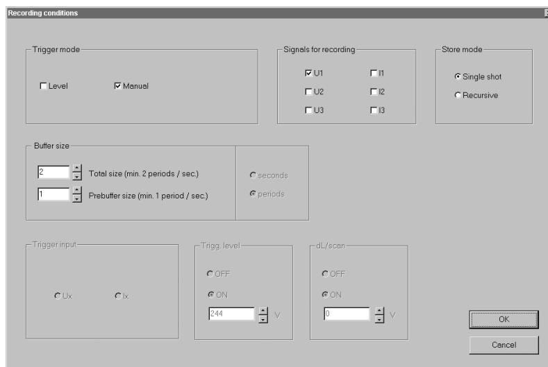
Fig. 29c: Ecran Détails pour enregistrement de phénomènes transitoires
