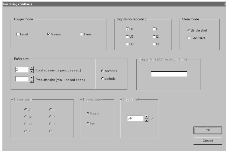
Fig. 29b: Ecran Détails pour enregistrement de formes d'ondes et d'enregistrement rapide
