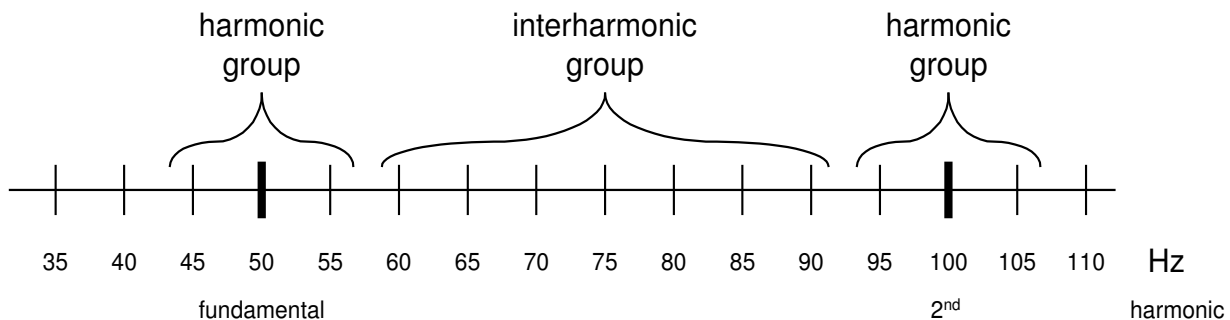
Fig. 15a: Détail d'un spectre d'interharmoniques
